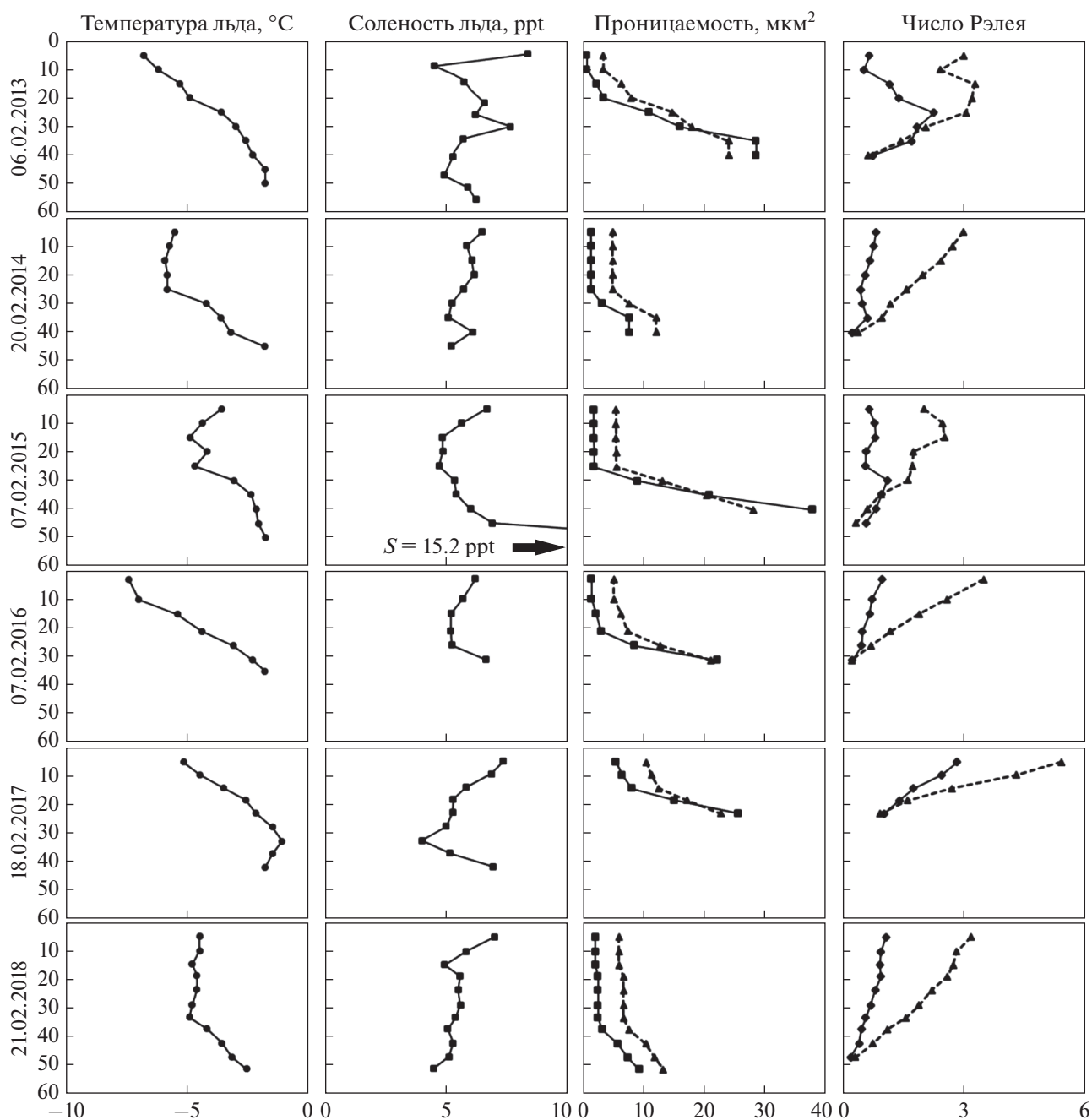
Рис. 1. Вертикальные профили температуры, солёности, проницаемости и числа Рэлея льда Амурского залива за период с 2013 по 2018 гг. Прерывистой линией обозначены результаты расчетов с учетом газовых включений.
