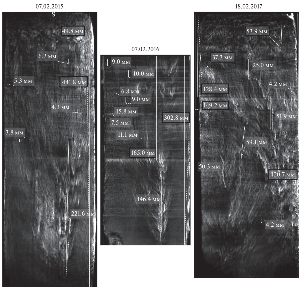
Рис. 3. МРТ-изображения кернов льда Амурского залива, взятых в 2015–2017 гг.
