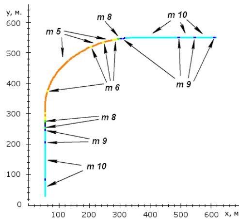
Рис. 2. Траектория движения объекта и соответствующие ей значения t
